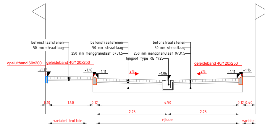
voorstel A-A V-profiel optie 1
