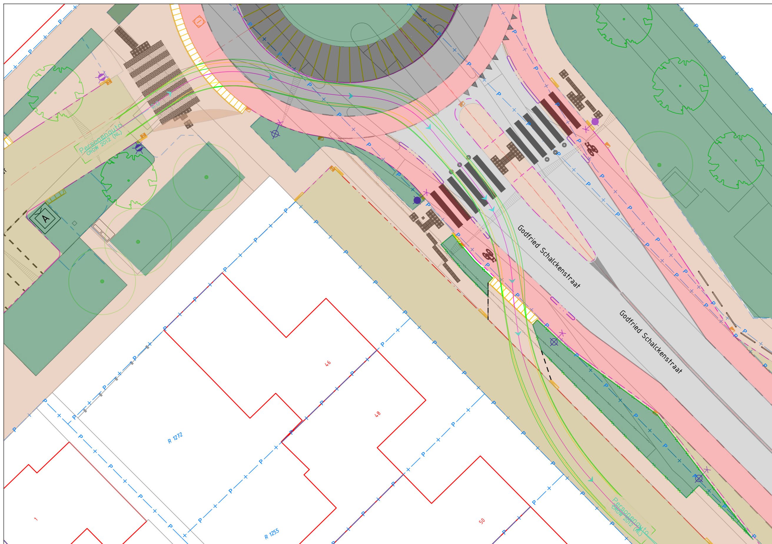
Uitsnede doorsteek Rotonde Made Blad 002 Schaal 1:200
